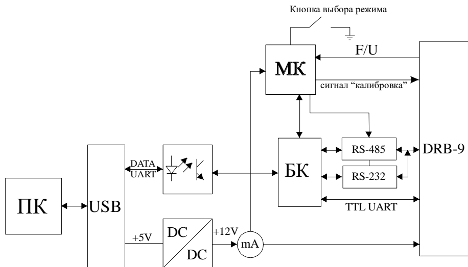
Рис. 3.3. Функциональная схема прибора
